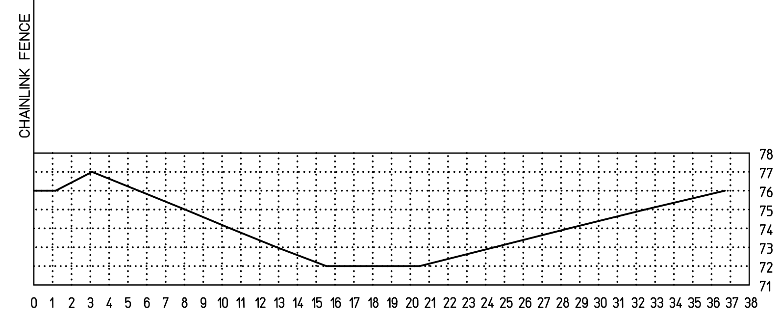
SECTION - A Scale: 1"=5'
