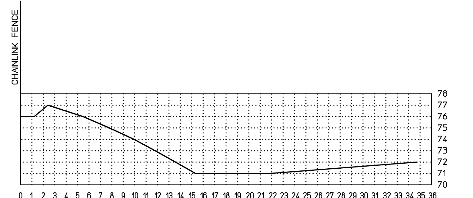
SECTION - B Scale: 1"=5'
